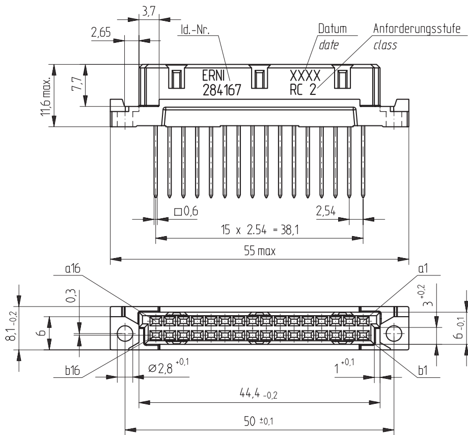
Bestückungsplan / contact layout
