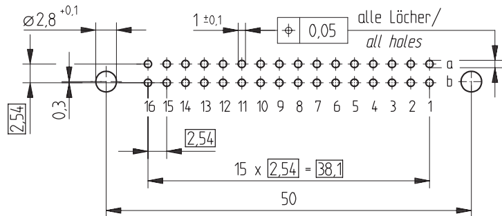
Leiterplatten-Lochbild / PCB drillhole pattern
