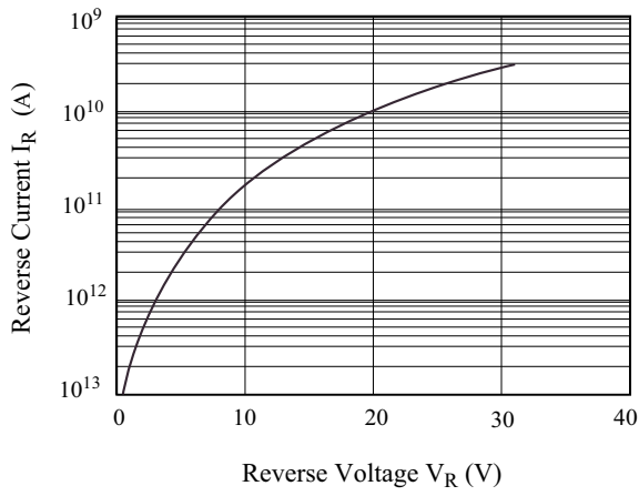
I_R - V_R
