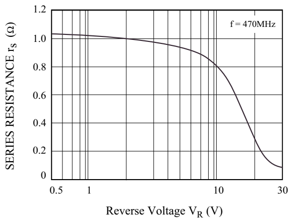
r_s - V_R
