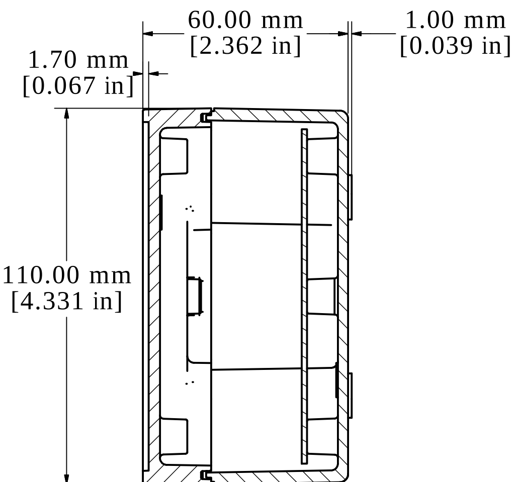
SECTION A-A
