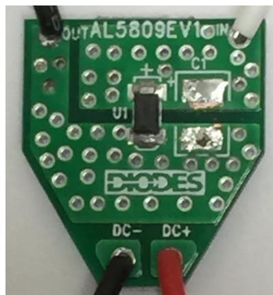
AL5809EV1 (PDI123)
