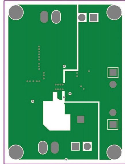
Fig. 25 - Inner Layer 1
