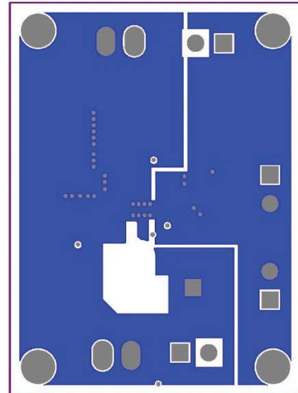
Fig. 26 - Bottom Layer
