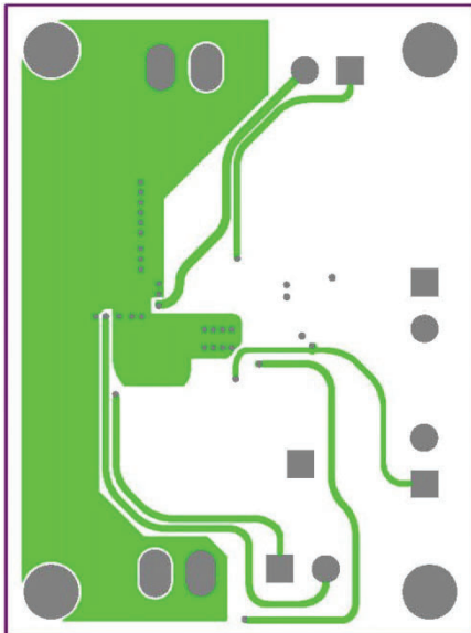
Fig. 24 - Inner Layer 2
