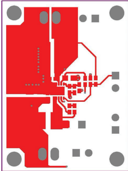
Fig. 23 - Top Layer
