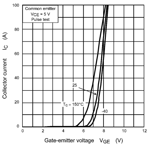
Fig. 8.5 I_C - V_{GE}
