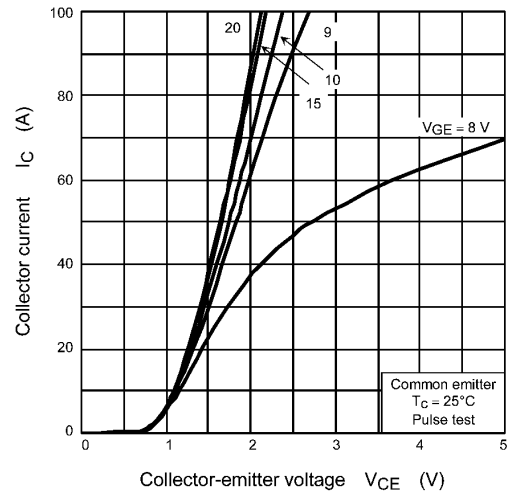
Fig. 8.2 I_C - V_{CE}
