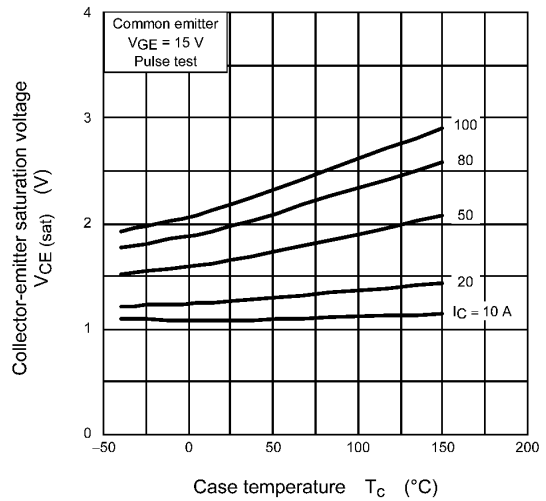
Fig. 8.4 V_{CE(sat)} - T_C
