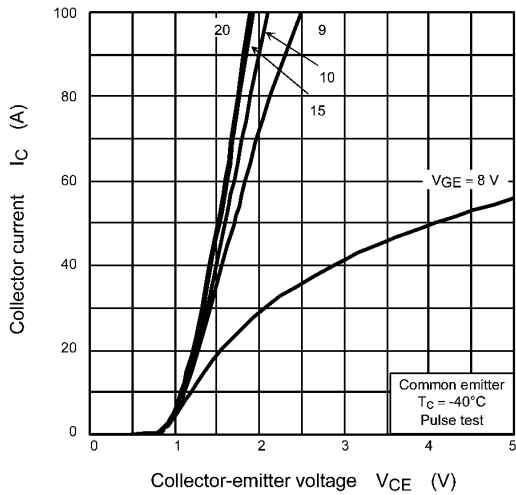
Fig. 8.1 I_C - V_{CE}
