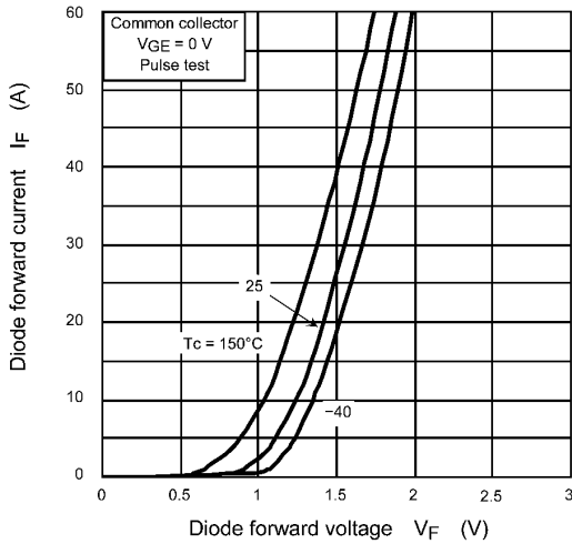
Fig. 8.13 I_F - V_F
