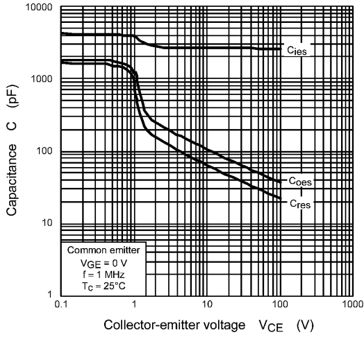
Fig. 8.7 C - V_{CE}
