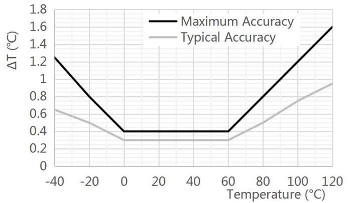
Figure2 温度 精度偏差
