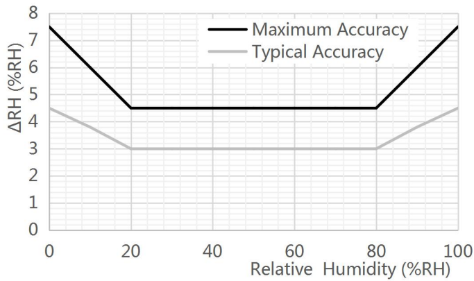
Figure 1 相对湿度 精度偏差
